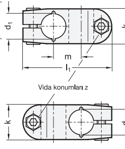
Altıgen somun
